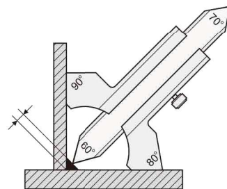
角焊缝测量 Angle Welds
