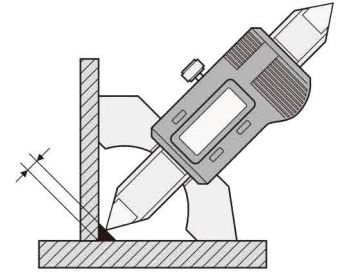
角焊缝测量 Angle Welds 0-20mm
