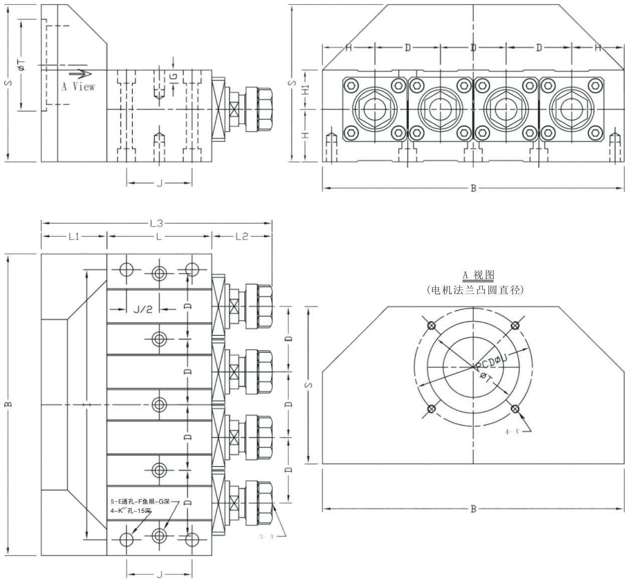
960-x40 四轴尺寸表：（实际尺寸依出货实物为准）
